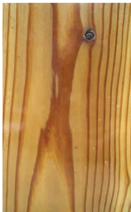
カラマツ材 屋外曝露 3 年間 塗膜の割れ・膨れ・剥がれ・ 白化等の劣化は見られない。
